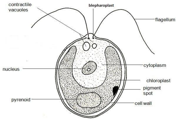
Chlamydomonas
